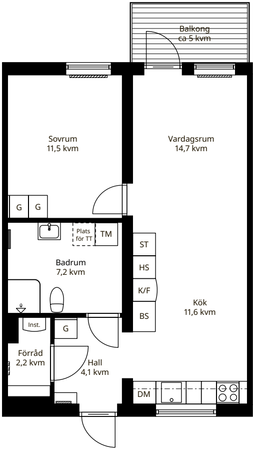
Rätvänd planlösning, skala 1:100
