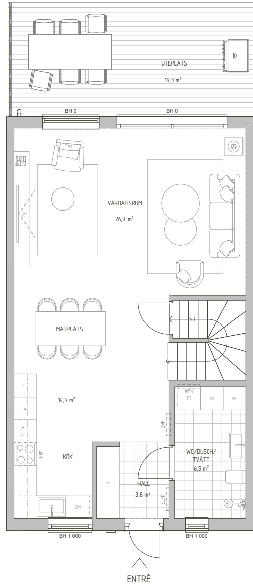
Entréplan
