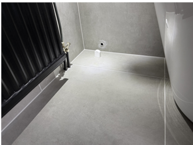
Rör i golv och vägg i våtzon 1 i plats för bad
